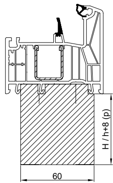
REHAU SYNEGO NV027
