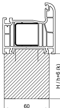
AVANTGARDE 7000 NV044
