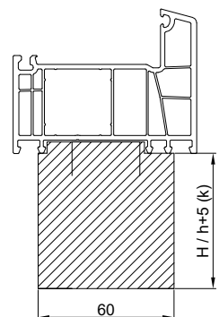
DECCO 82 NV046
